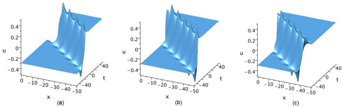
Fig. 1 – Kinky breather wave solution (8): a) y = -2 ; b) y = 0 ; c) y = 3 .
